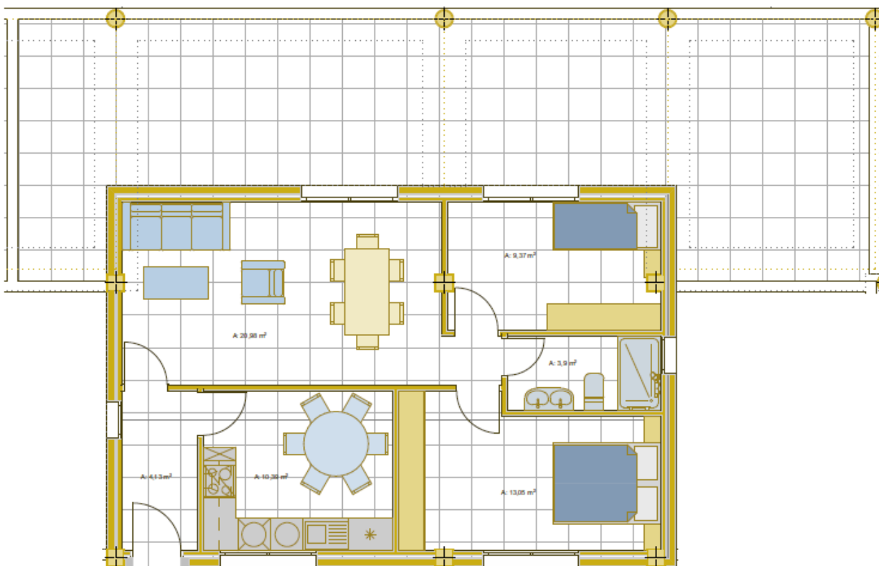
PLANTA ATICO
